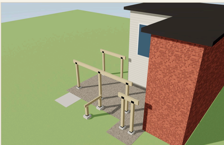
Step 4 · Beams — DROP (2)2x10 SYP N (2 posts) · DROP (2)2x10 SYP N+S (3 posts) · DROP (2)2x10 SYP L (2 posts)
